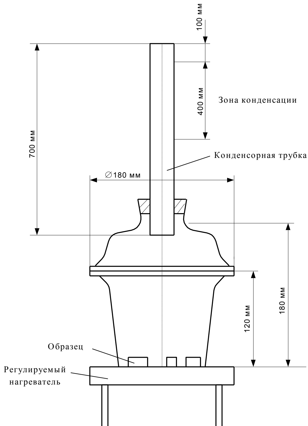
Рисунок 6.1 - Пример кипятивника для испытаний на диффузию воды
